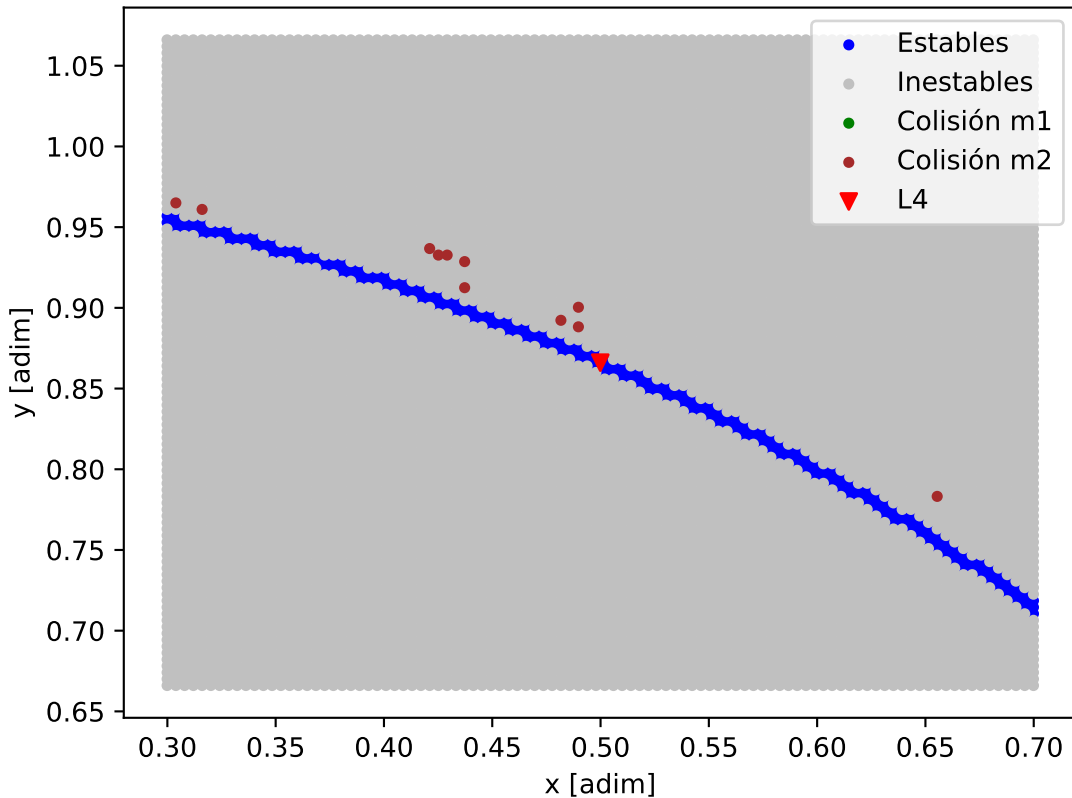
Mapa de estabilidad - HD_156668
