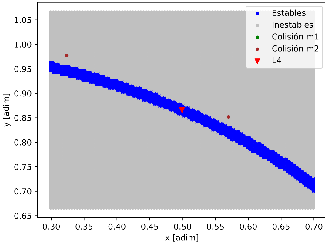
Mapa de estabilidad - HD_202696
