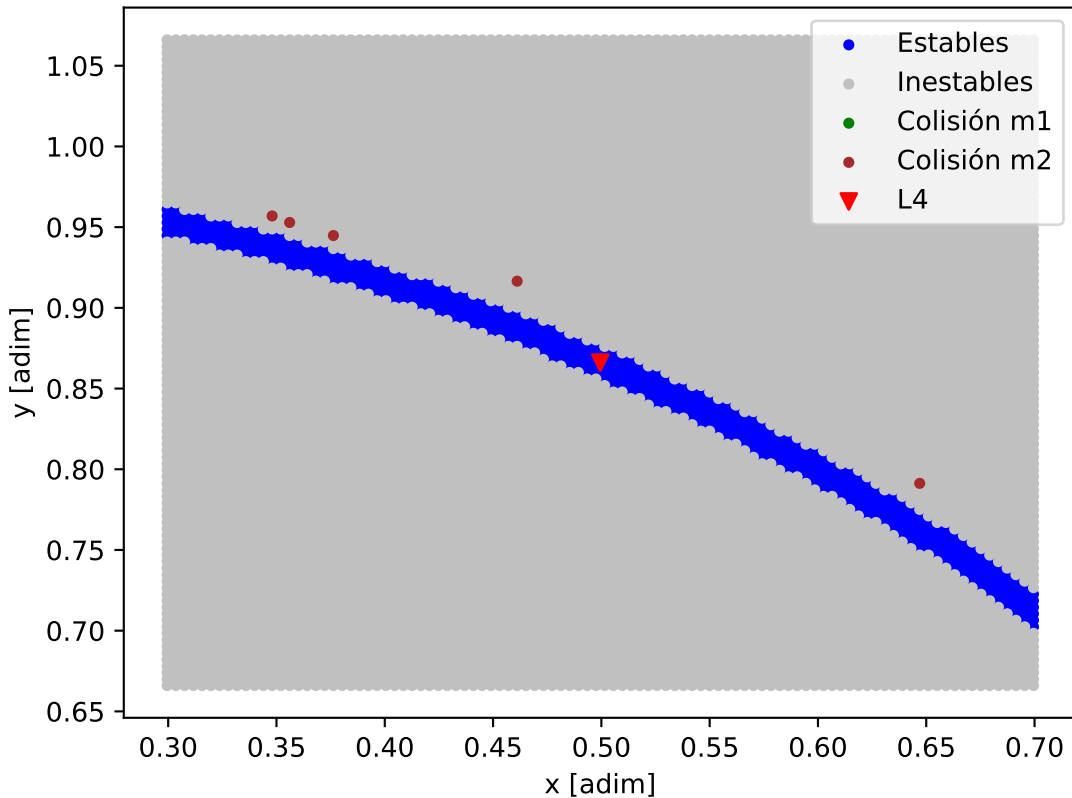
Mapa de estabilidad - HD_215497
