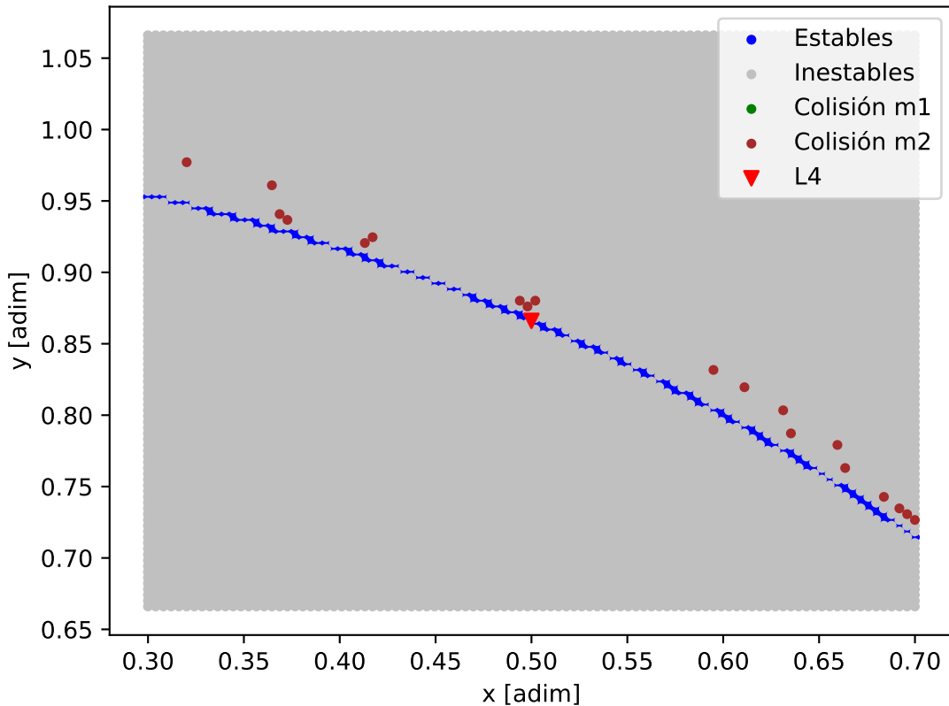
Mapa de estabilidad - HD_216520
