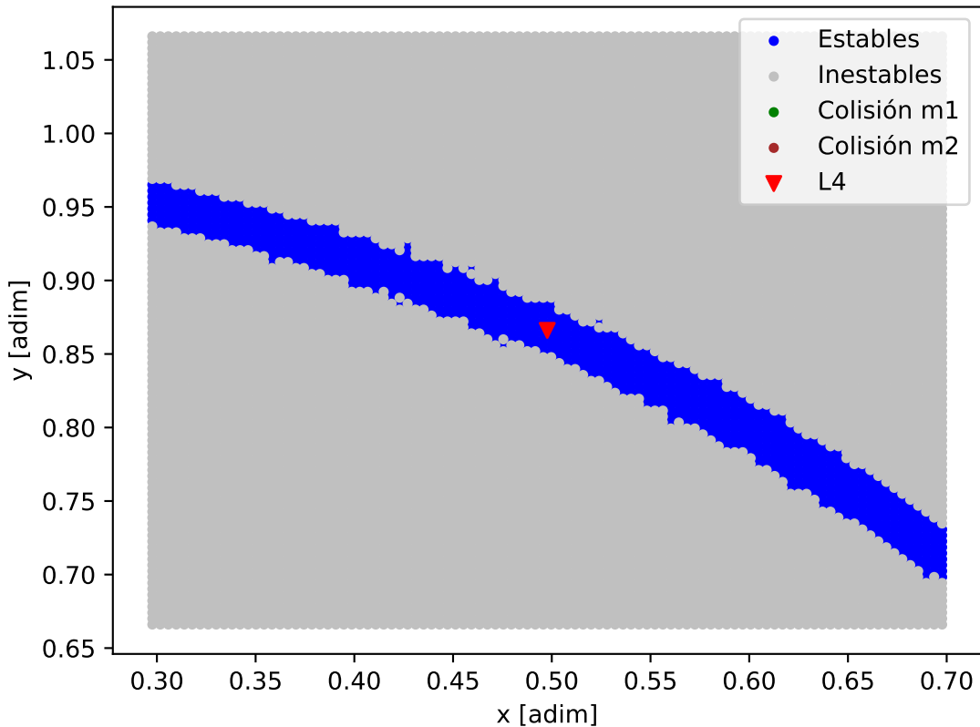
Mapa de estabilidad - HD_4732
