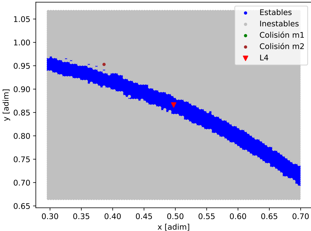
Mapa de estabilidad - HD_87816
