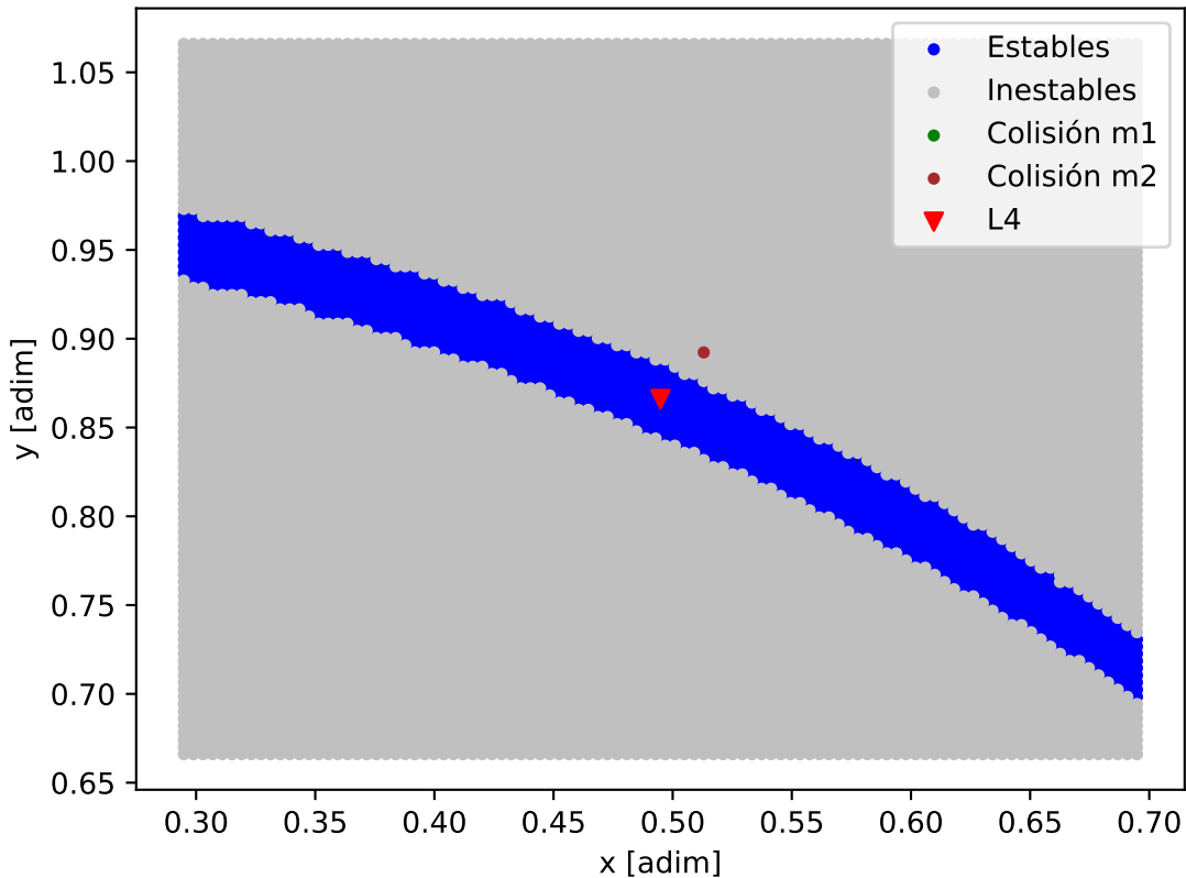
Mapa de estabilidad - HIP_67851
