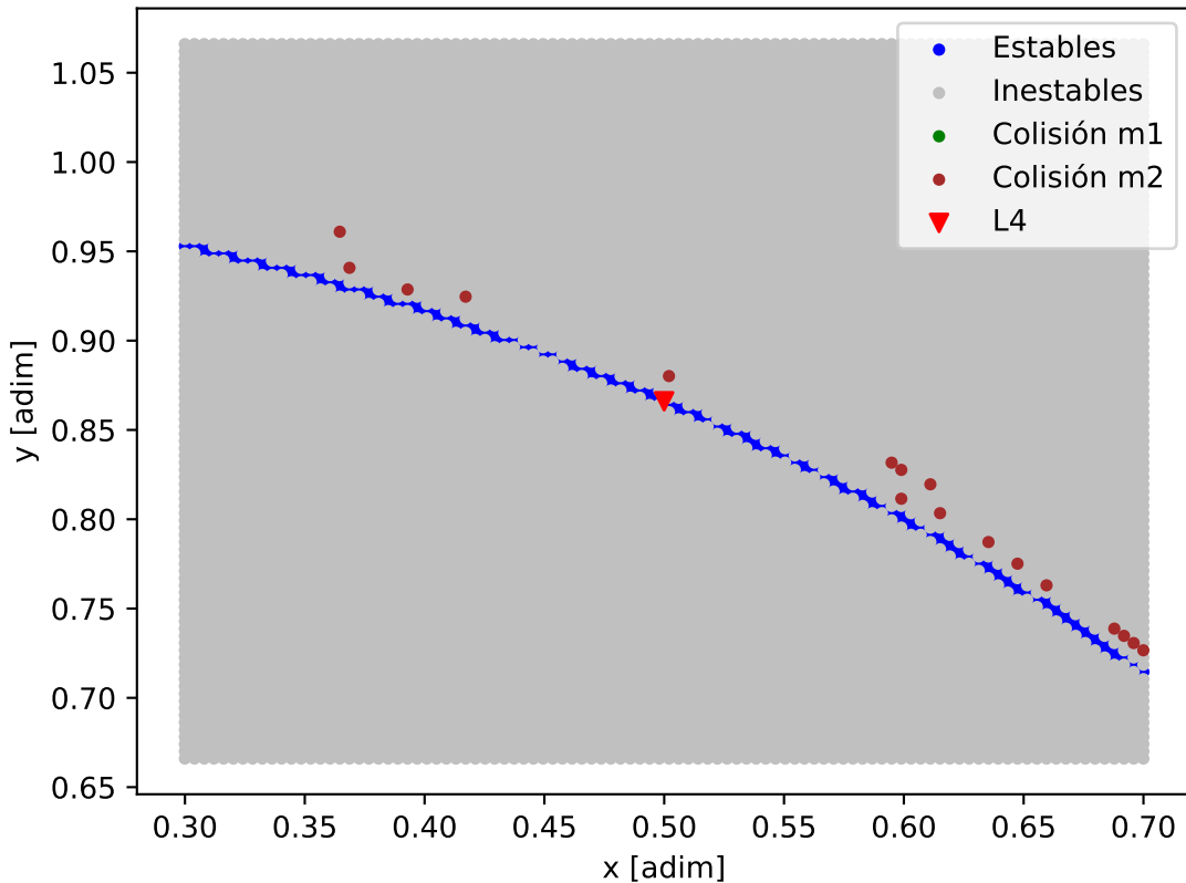
Mapa de estabilidad - K2-233
