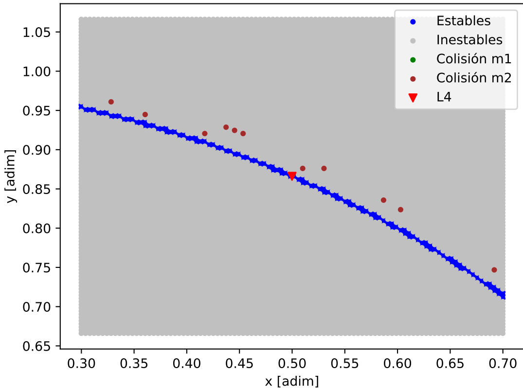
Mapa de estabilidad - Kepler-411
