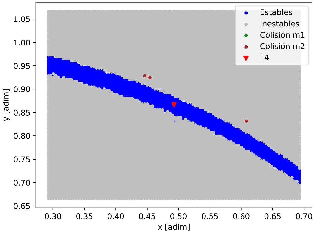
Mapa de estabilidad - PDS_70
