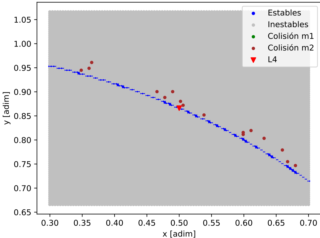
Mapa de estabilidad - TOI-1246
