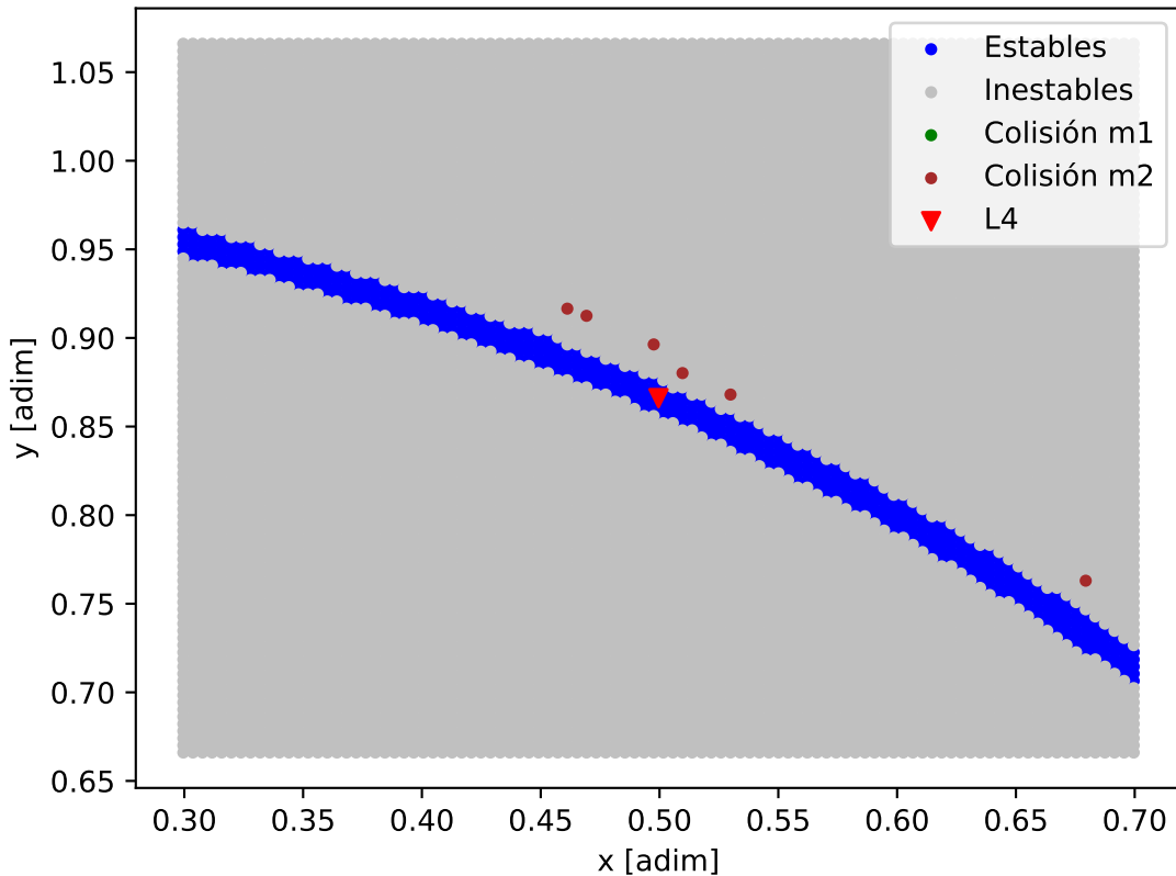
Mapa de estabilidad - TOI-2202
