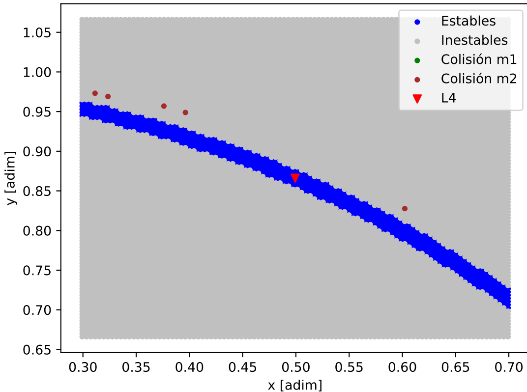
Mapa de estabilidad - TOI-2525
