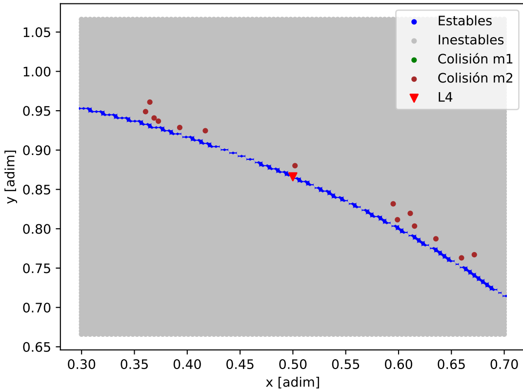
Mapa de estabilidad - TOI-969
