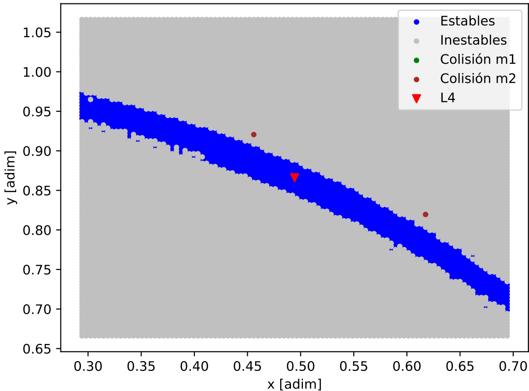
Mapa de estabilidad - TYC_8998-760-1
