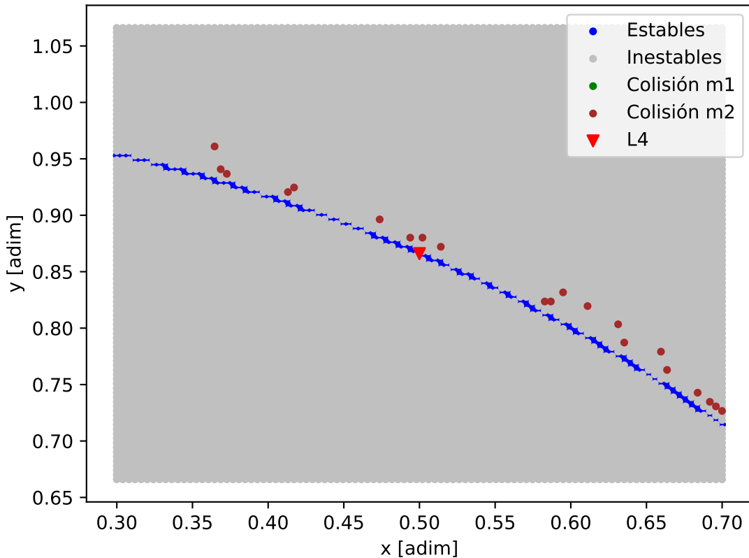
Mapa de estabilidad - GJ_1002
