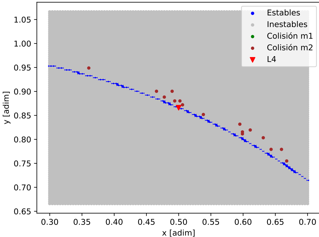
Mapa de estabilidad - GJ_1132
