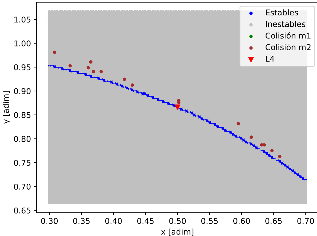
Mapa de estabilidad - GJ_180
