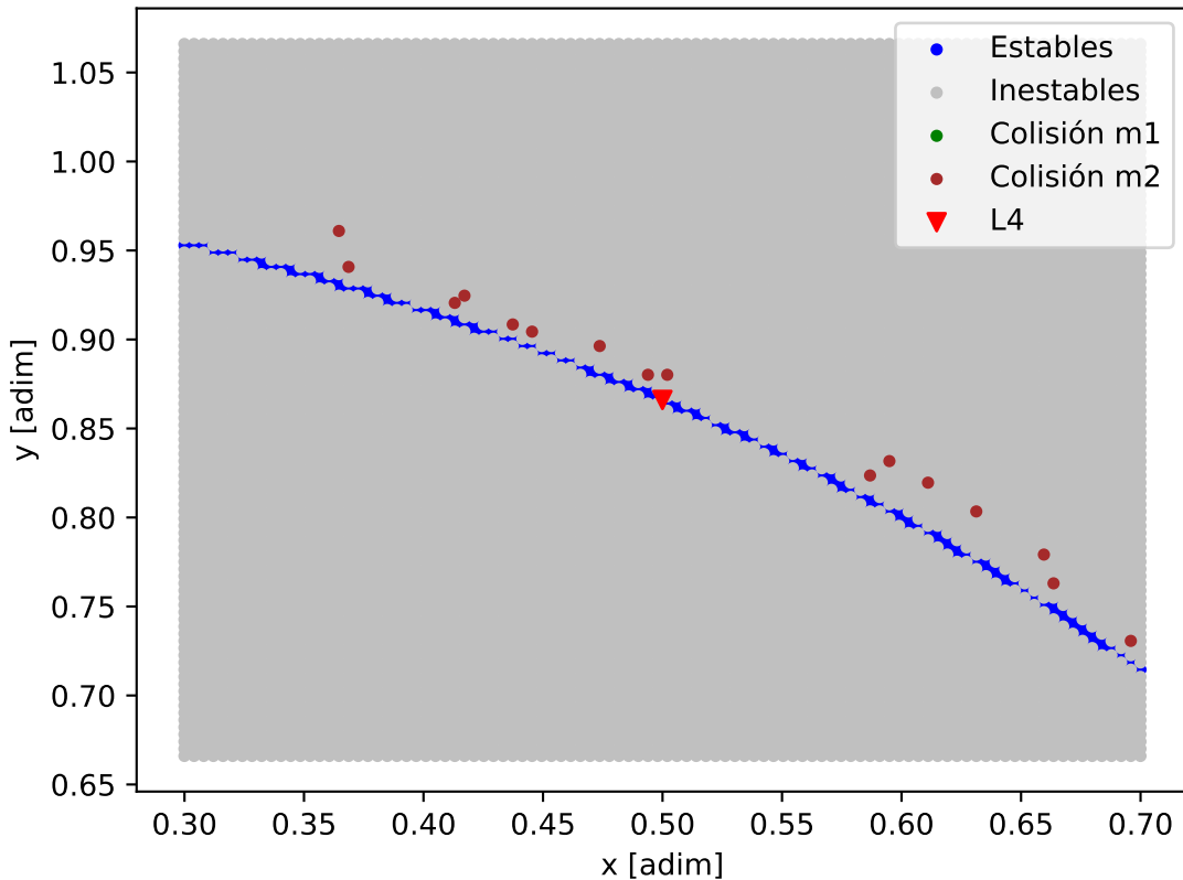
Mapa de estabilidad - GJ_251
