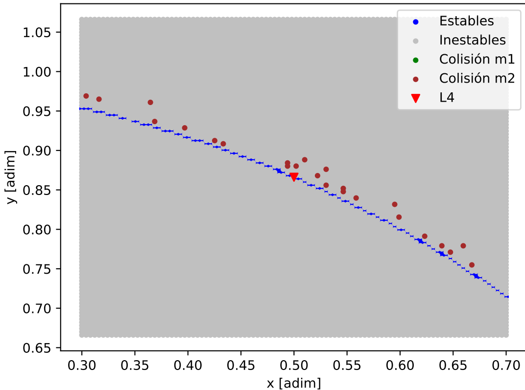
Mapa de estabilidad - GJ_3138
