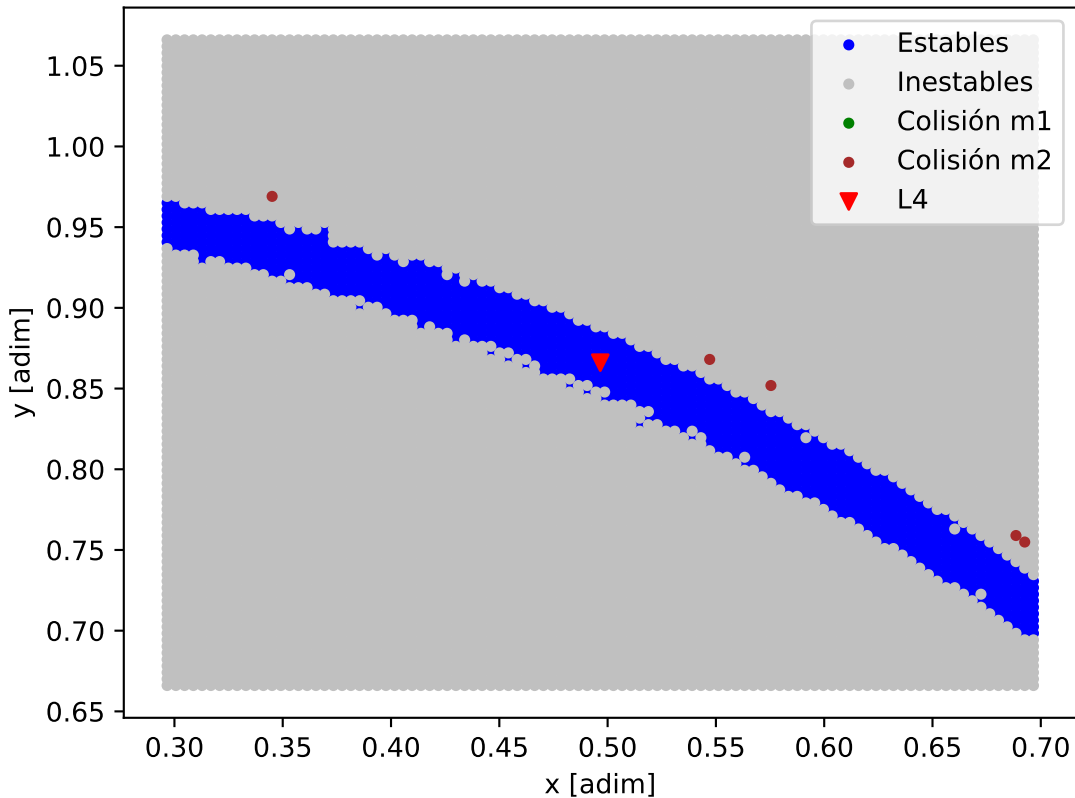
Mapa de estabilidad - GJ_317
