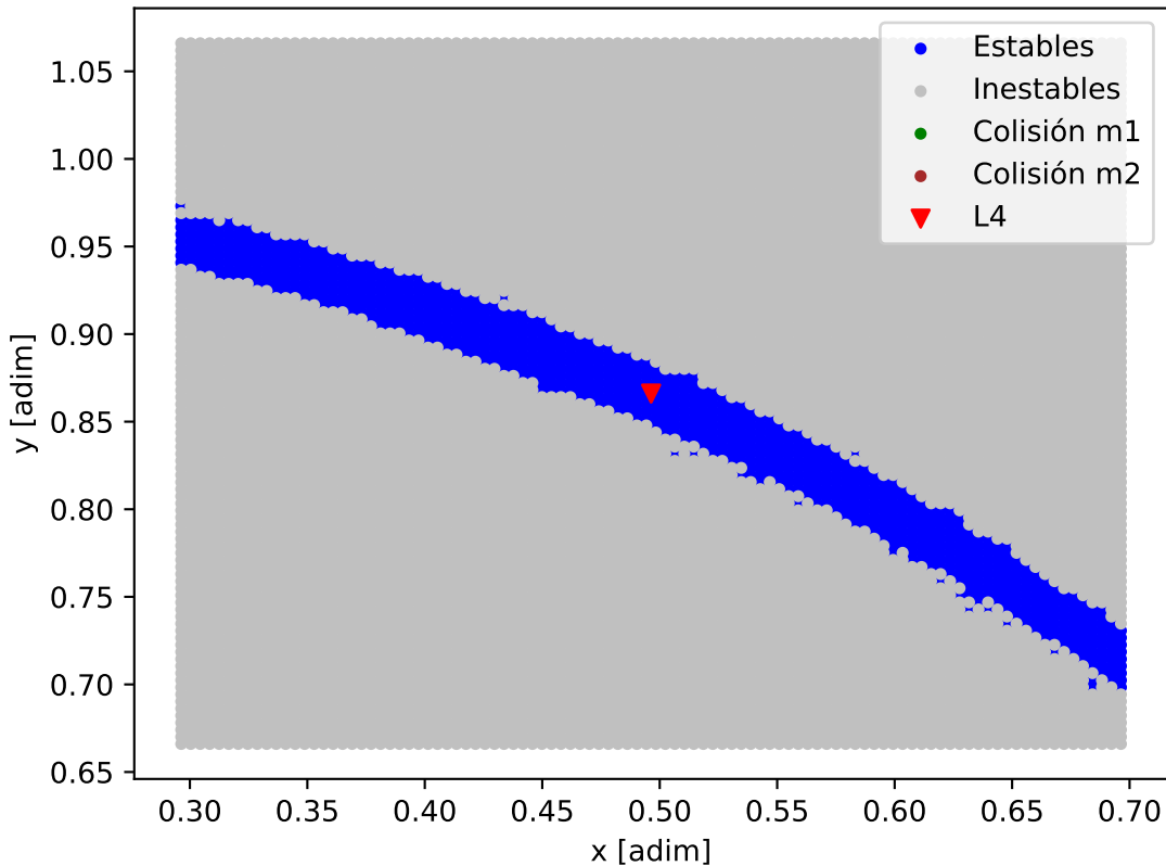
Mapa de estabilidad - GJ_328
