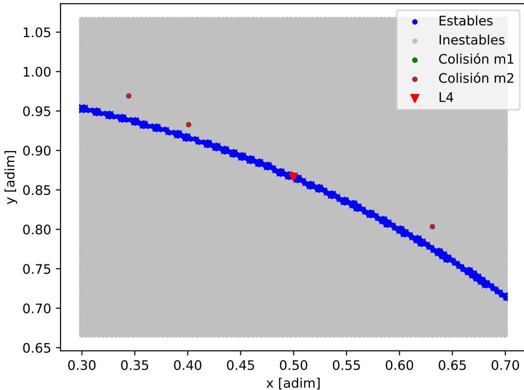
Mapa de estabilidad - GJ_3293
