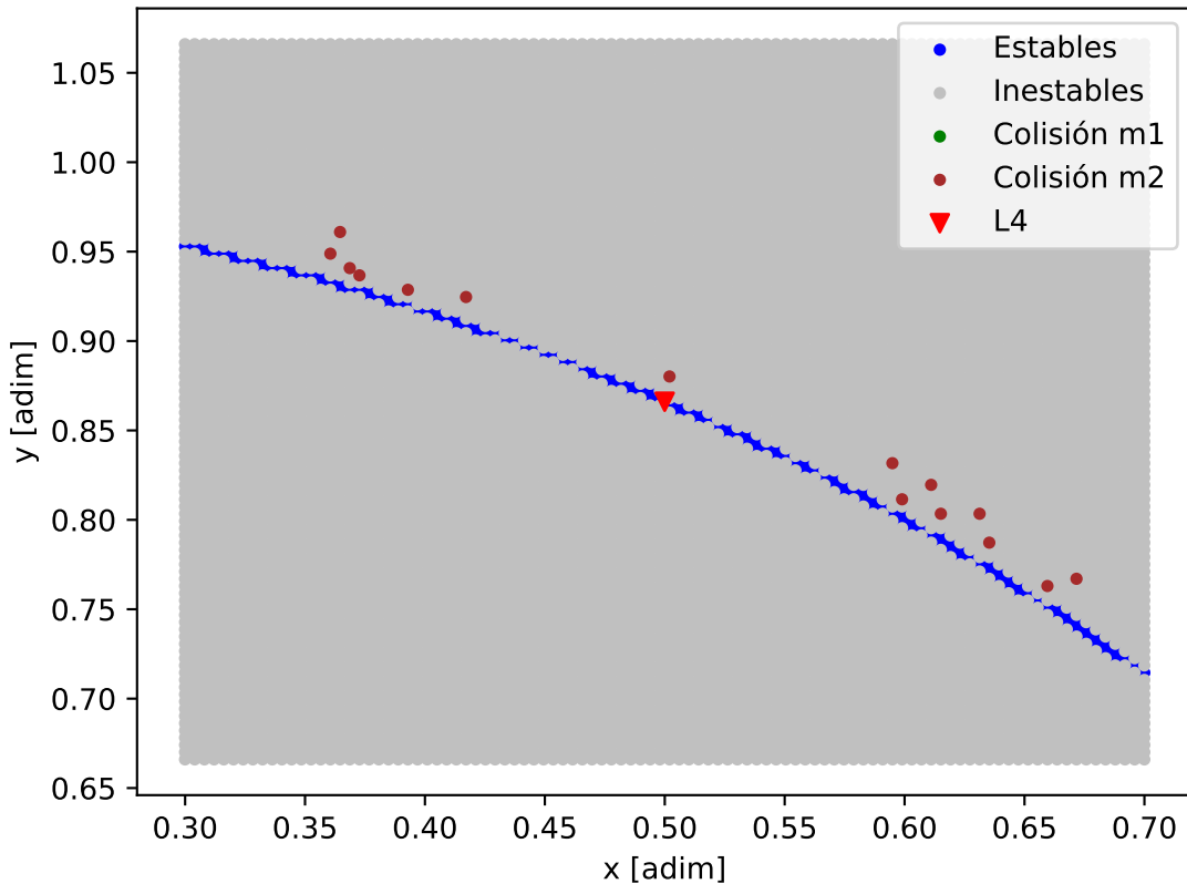
Mapa de estabilidad - GJ_3323
