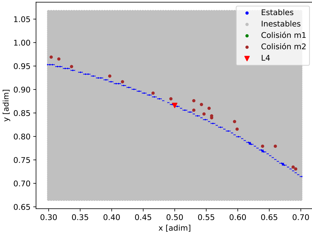
Mapa de estabilidad - GJ_3929
