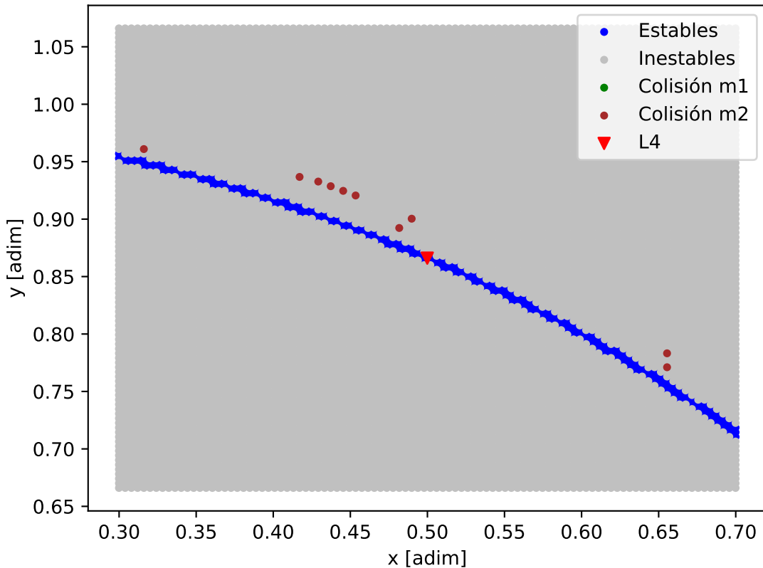
Mapa de estabilidad - GJ_411
