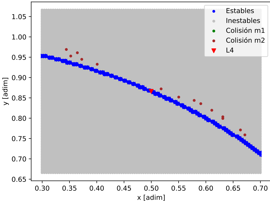
Mapa de estabilidad - GJ_433
