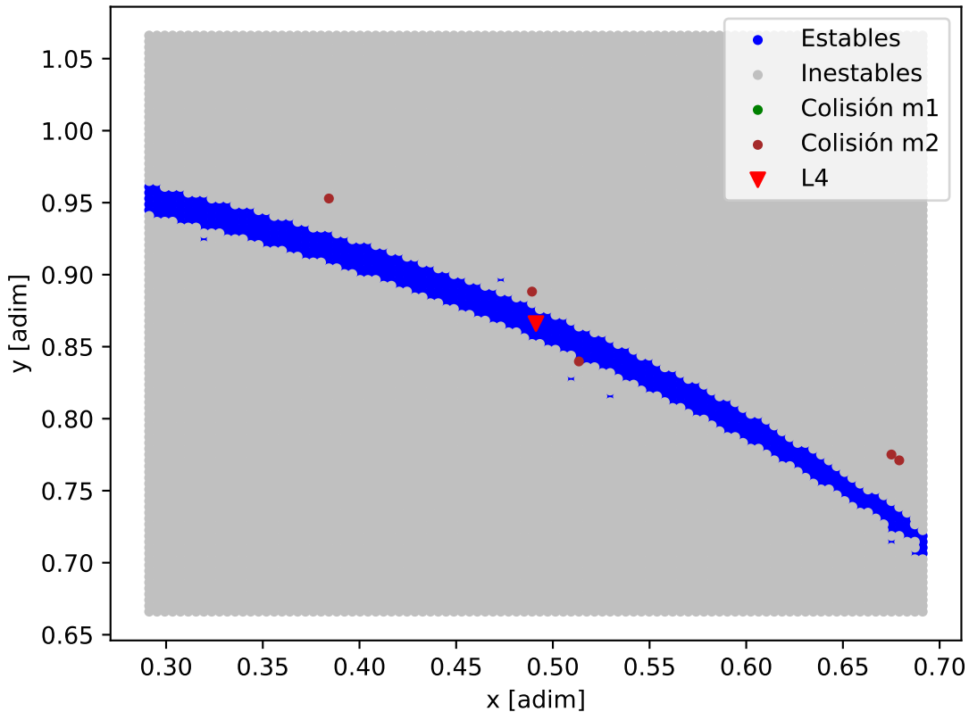
Mapa de estabilidad - GJ_676_A
