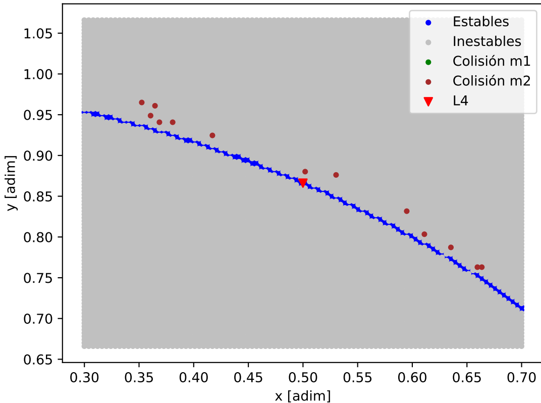
Mapa de estabilidad - GJ_682
