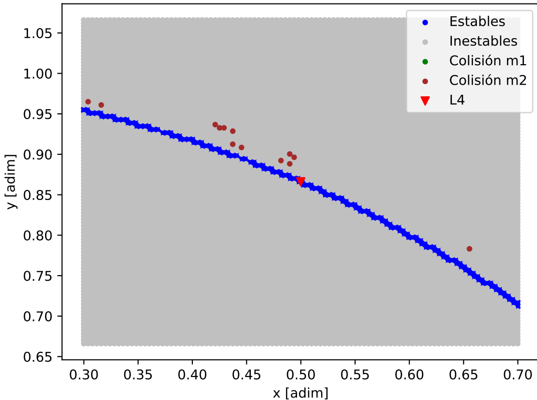
Mapa de estabilidad - GJ_687
