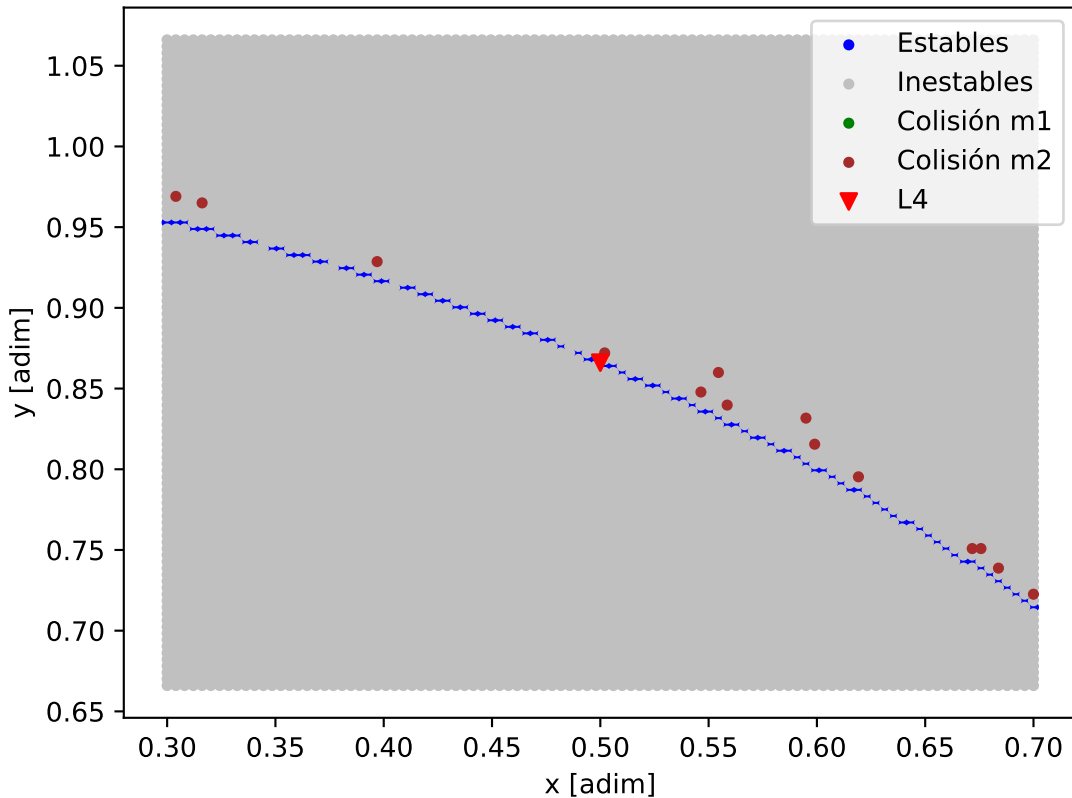
Mapa de estabilidad - GJ_806
