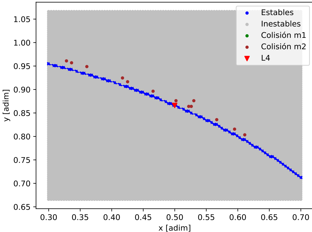
Mapa de estabilidad - GJ_876
