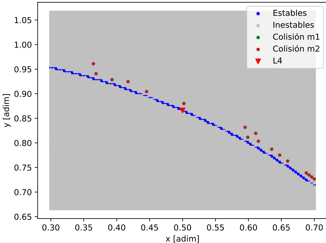
Mapa de estabilidad - GJ_887
