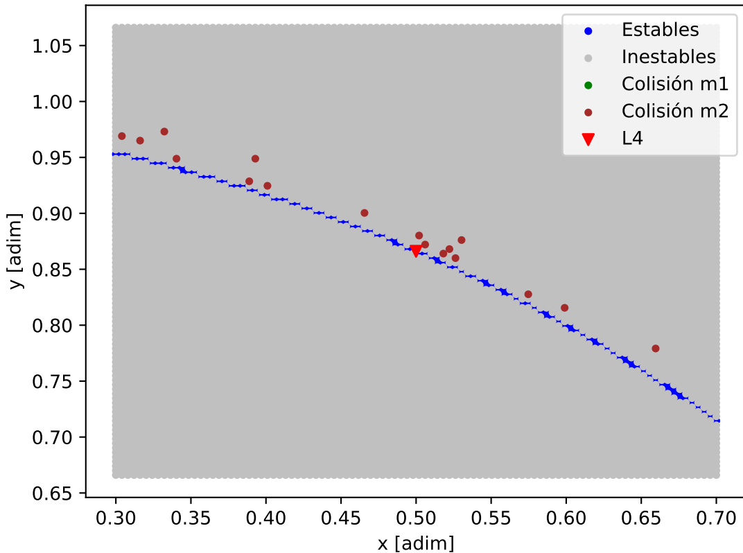
Mapa de estabilidad - G_192-15
