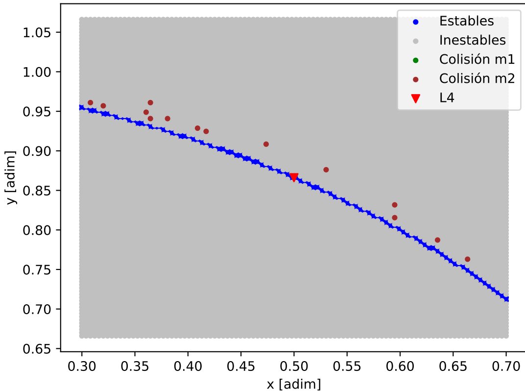
Mapa de estabilidad - K2-146
