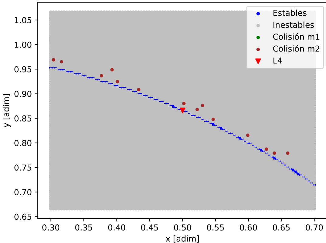
Mapa de estabilidad - K2-154
