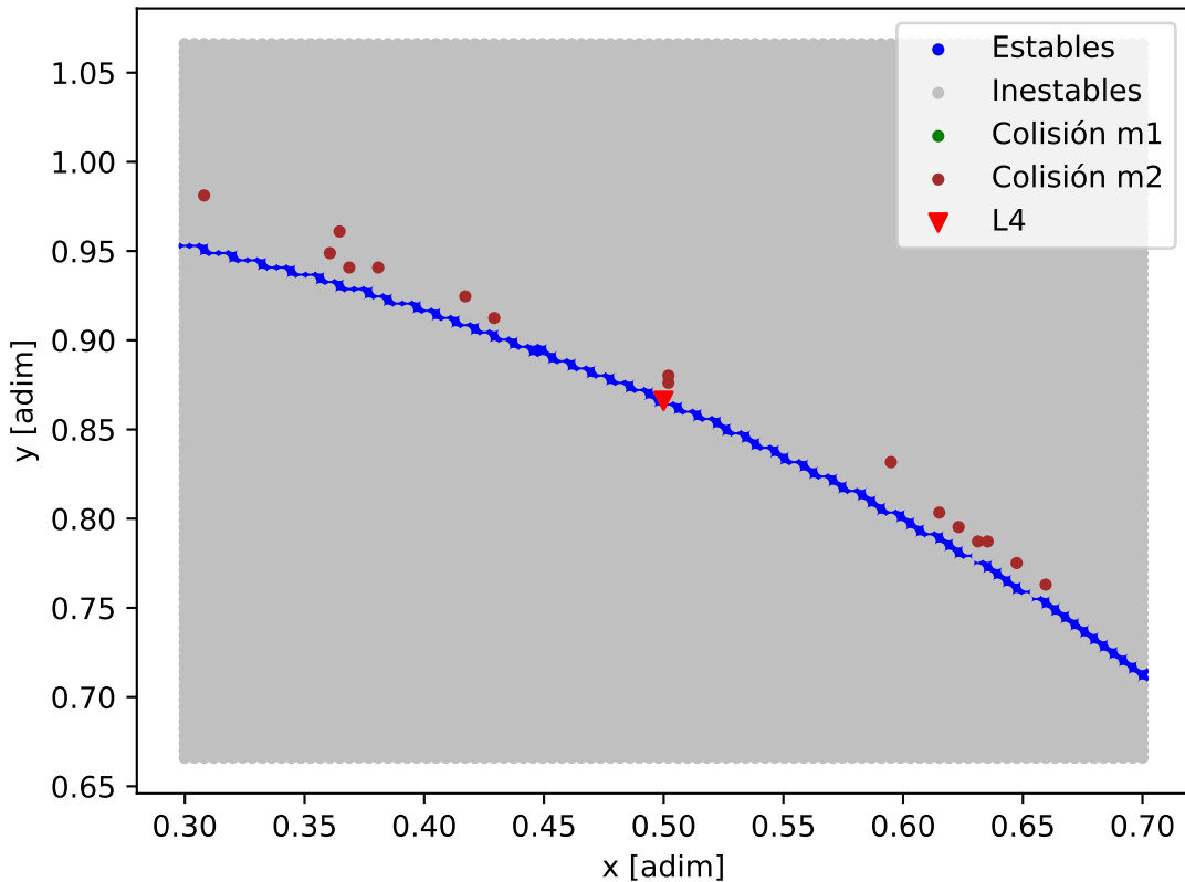
Mapa de estabilidad - K2-264
