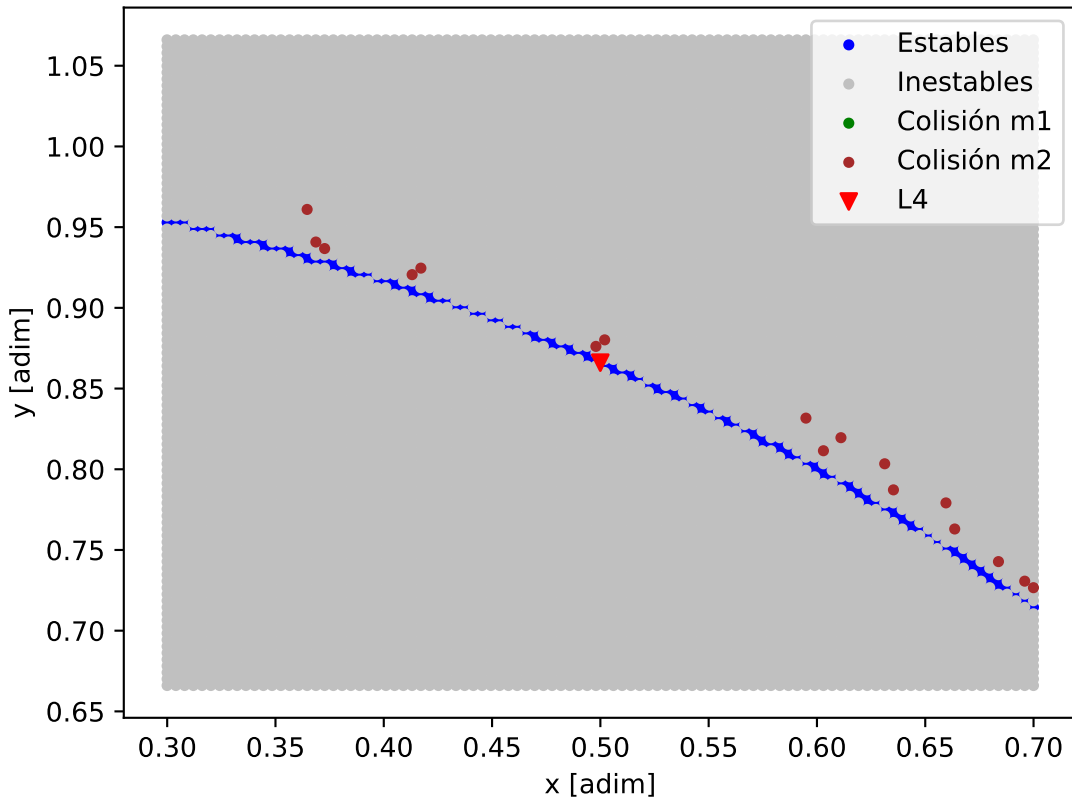
Mapa de estabilidad - Kepler-26
