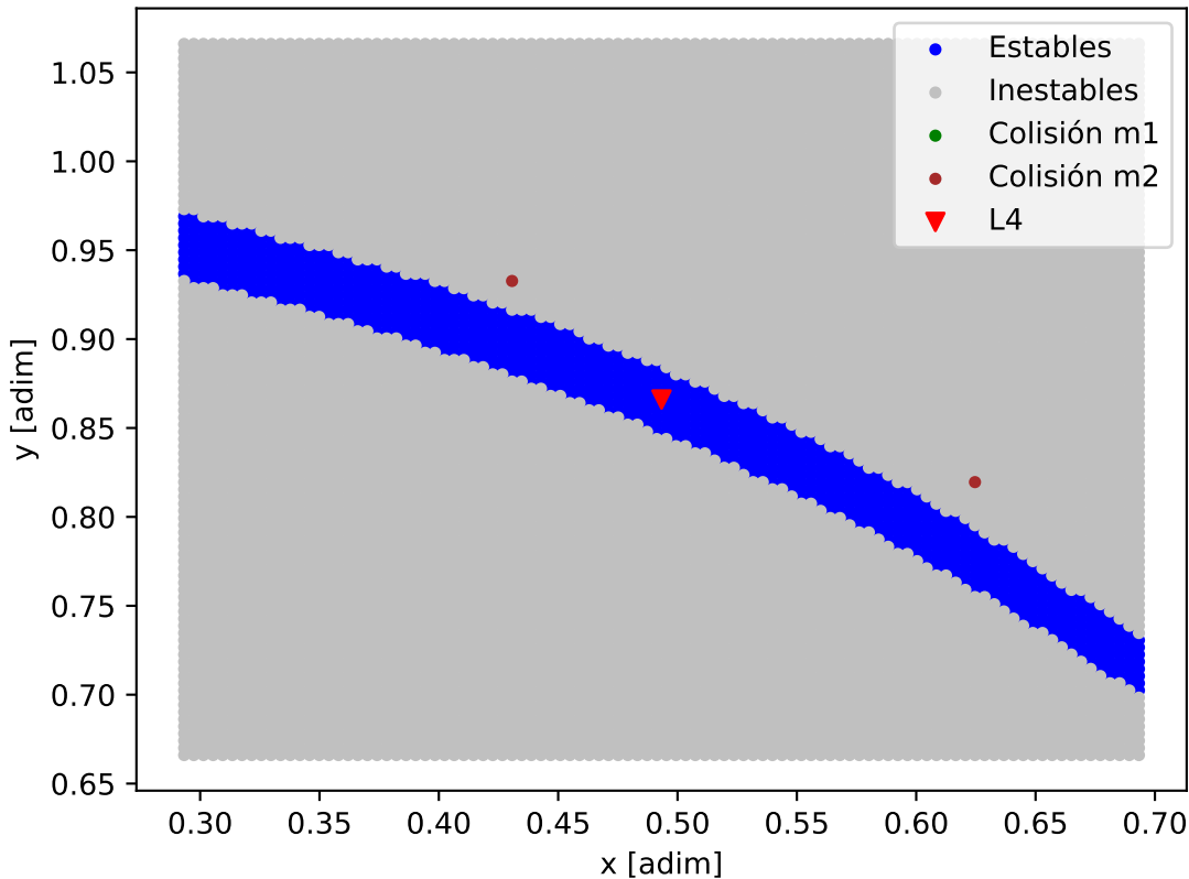
Mapa de estabilidad - Kepler-32
