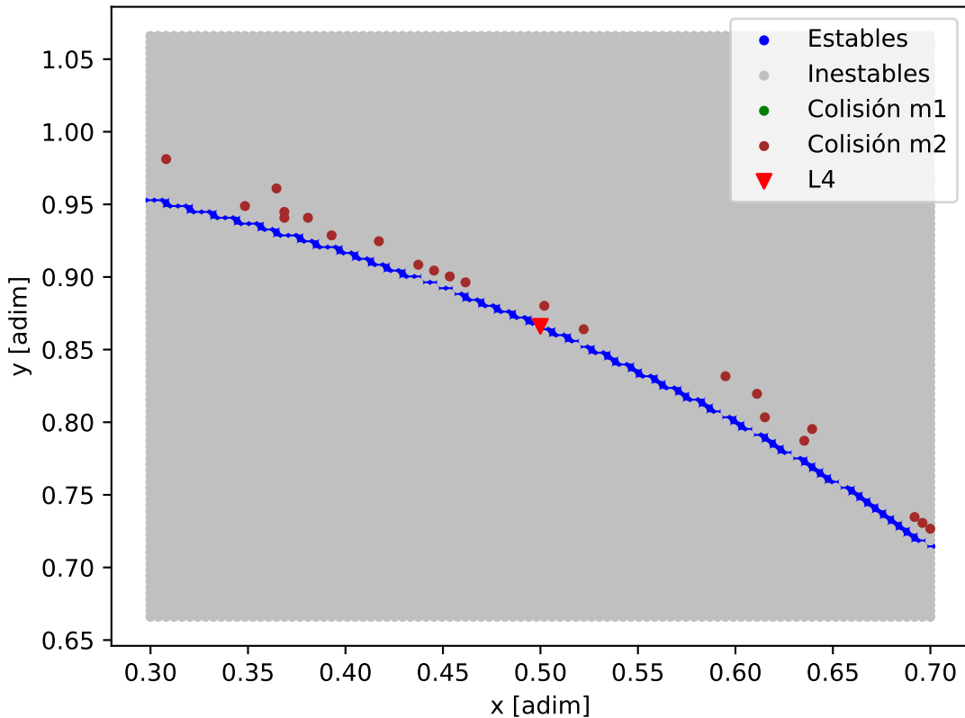
Mapa de estabilidad - Kepler-49
