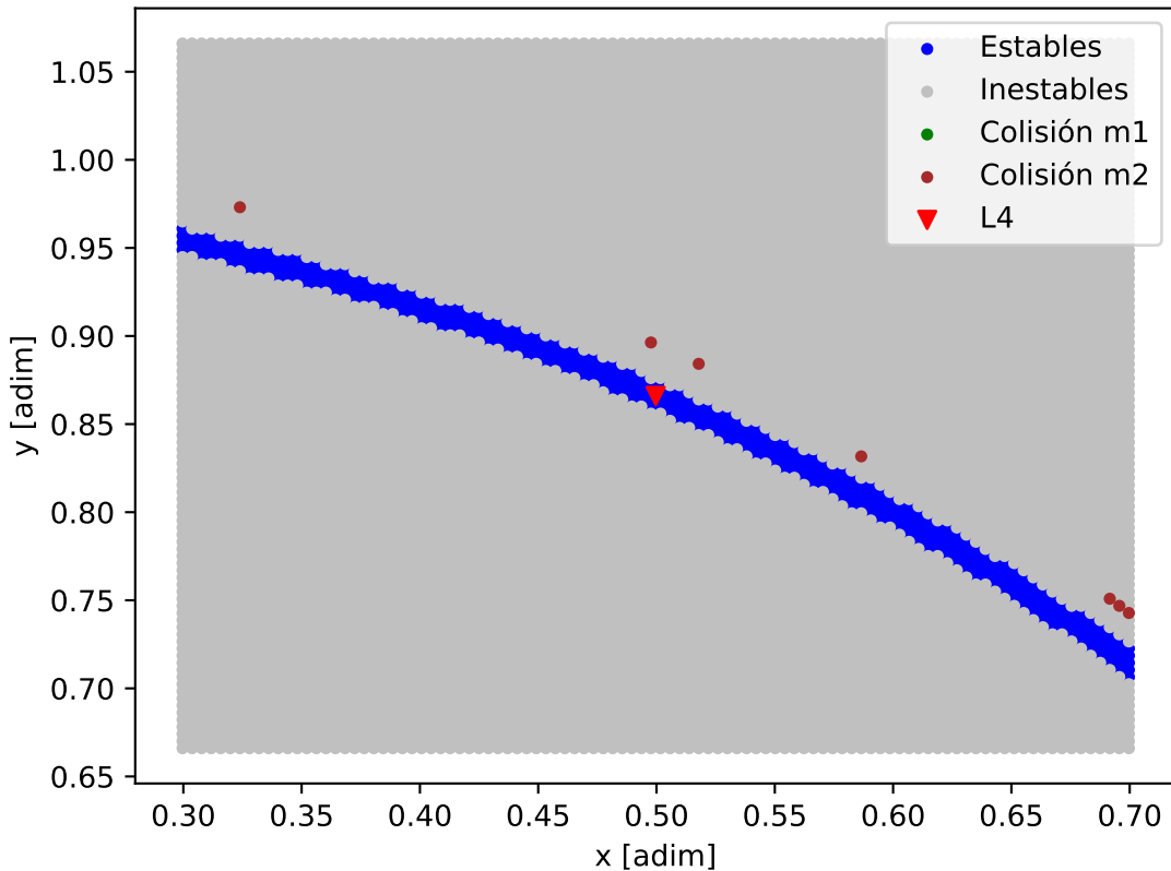
Mapa de estabilidad - LP_890-9
