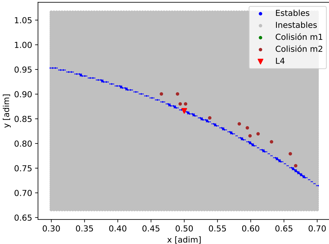
Mapa de estabilidad - L_98-59
