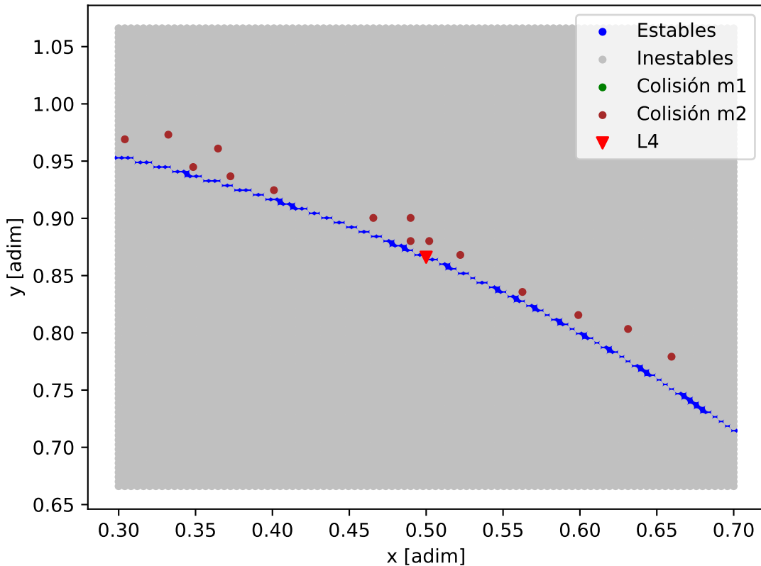
Mapa de estabilidad - TOI-1468
