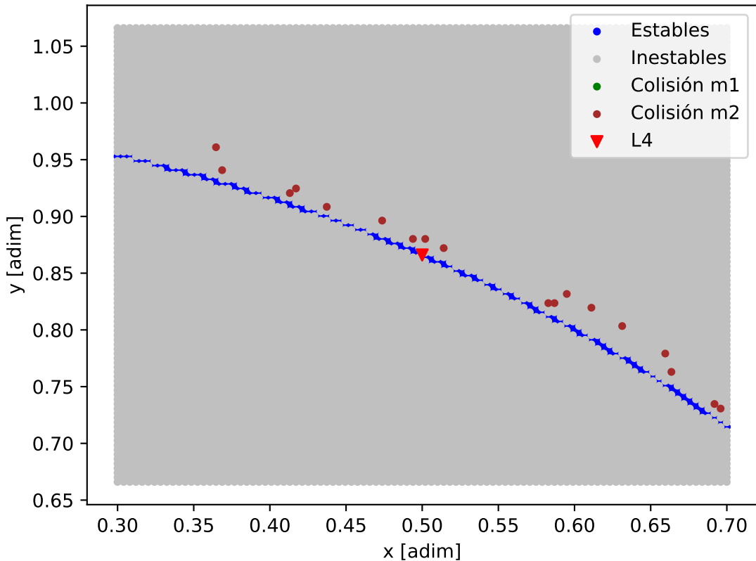
Mapa de estabilidad - TOI-1752
