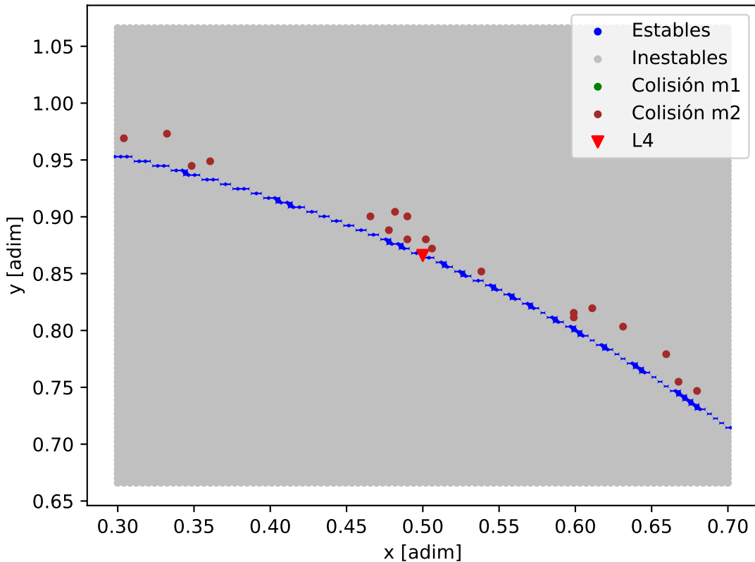
Mapa de estabilidad - TOI-2096
