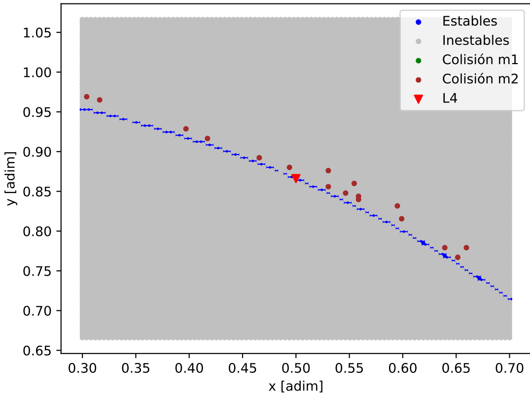
Mapa de estabilidad - TOI-2267_A
