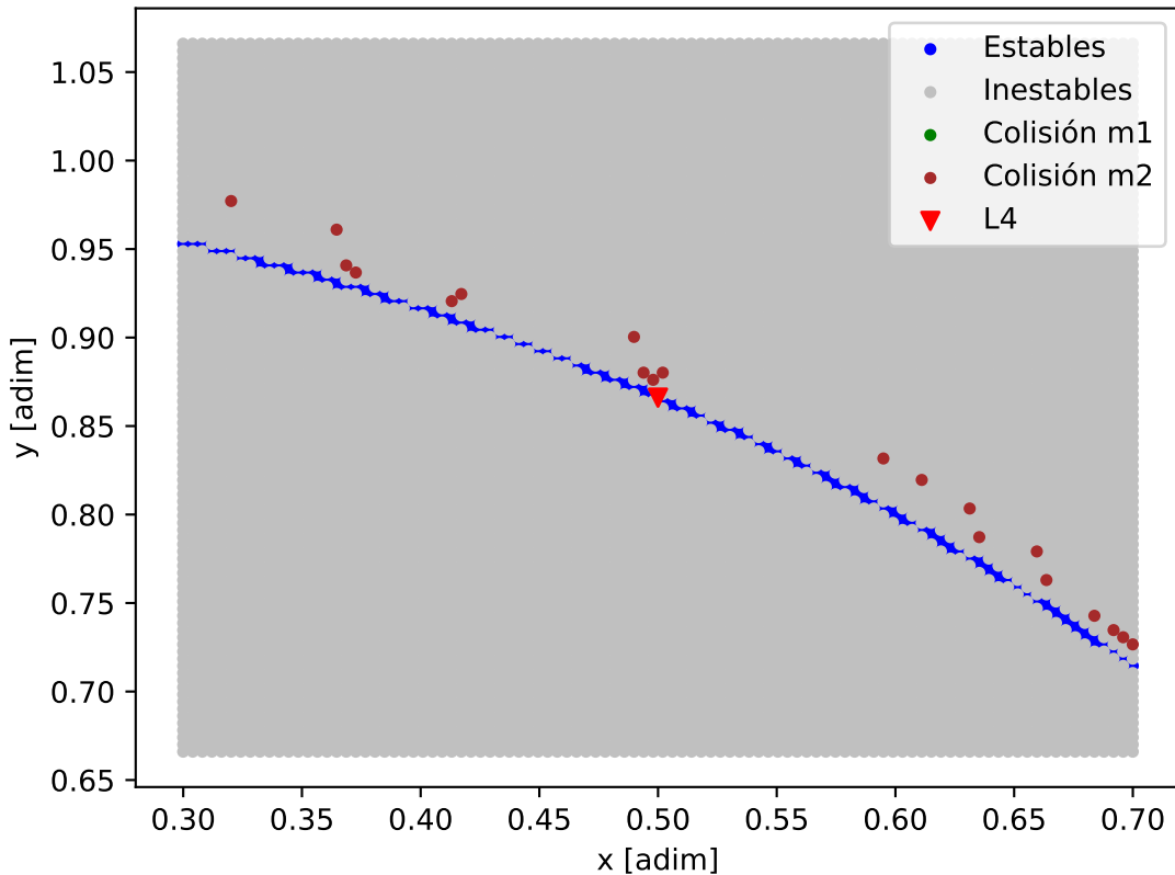
Mapa de estabilidad - TOI-5799
