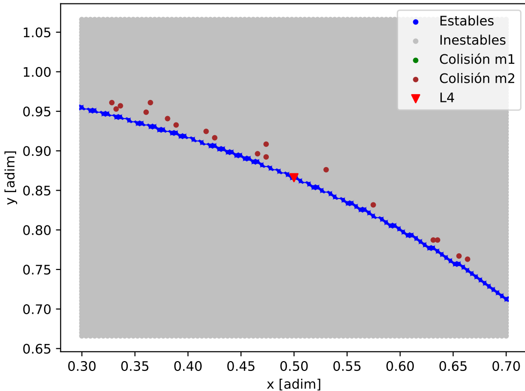
Mapa de estabilidad - TOI-756
