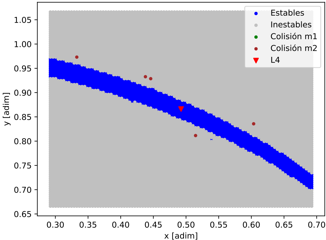
Mapa de estabilidad - TOI-756
