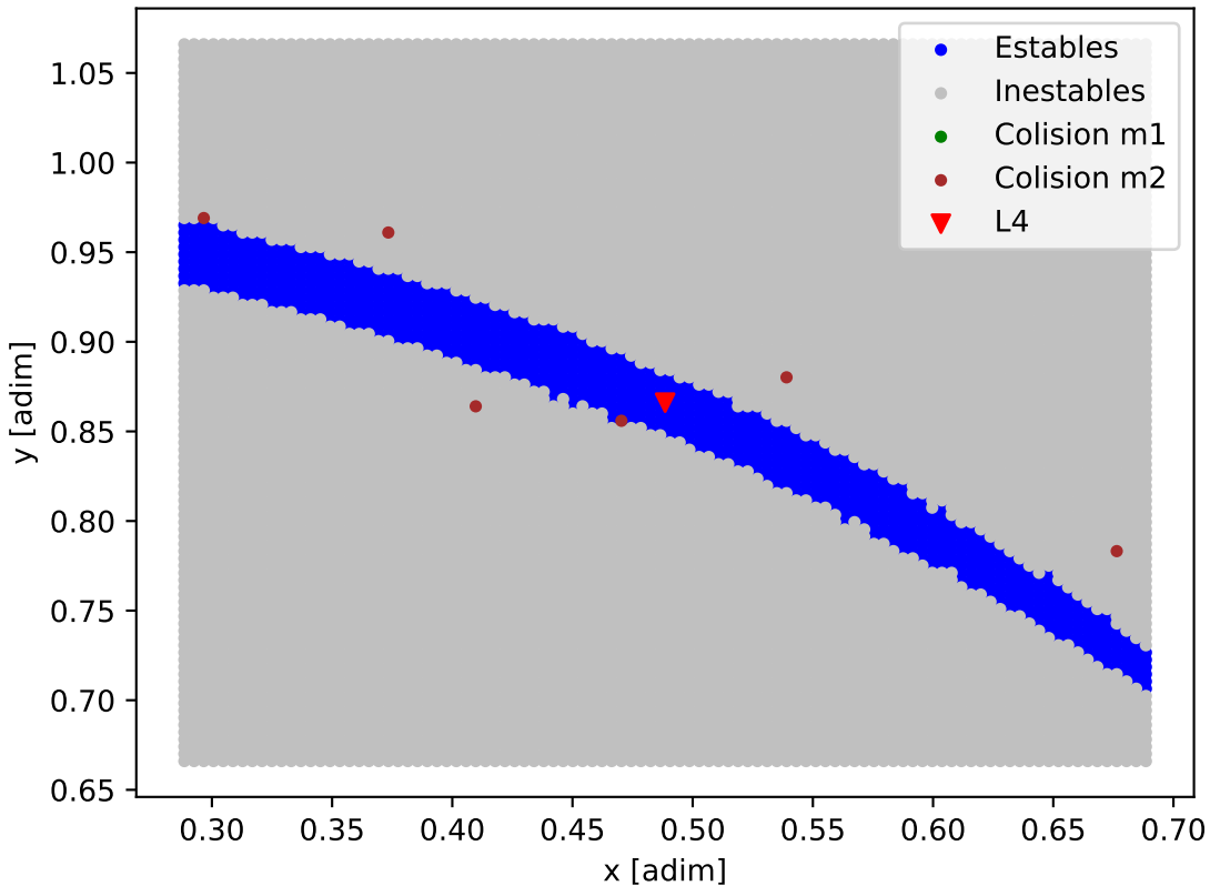
Mapa de estabilidad - HD_217786
